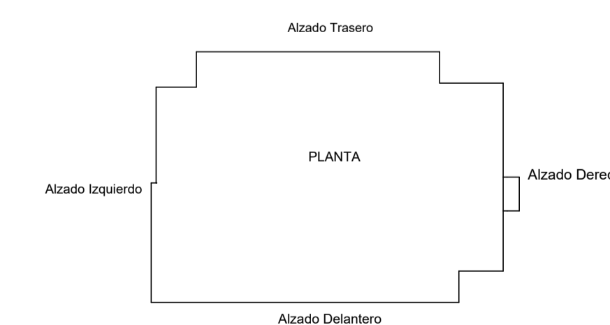
Alzado Derecho
